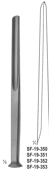
ALEXANDER SF-19-350 - SF-19-353 Gouges 170 mm
